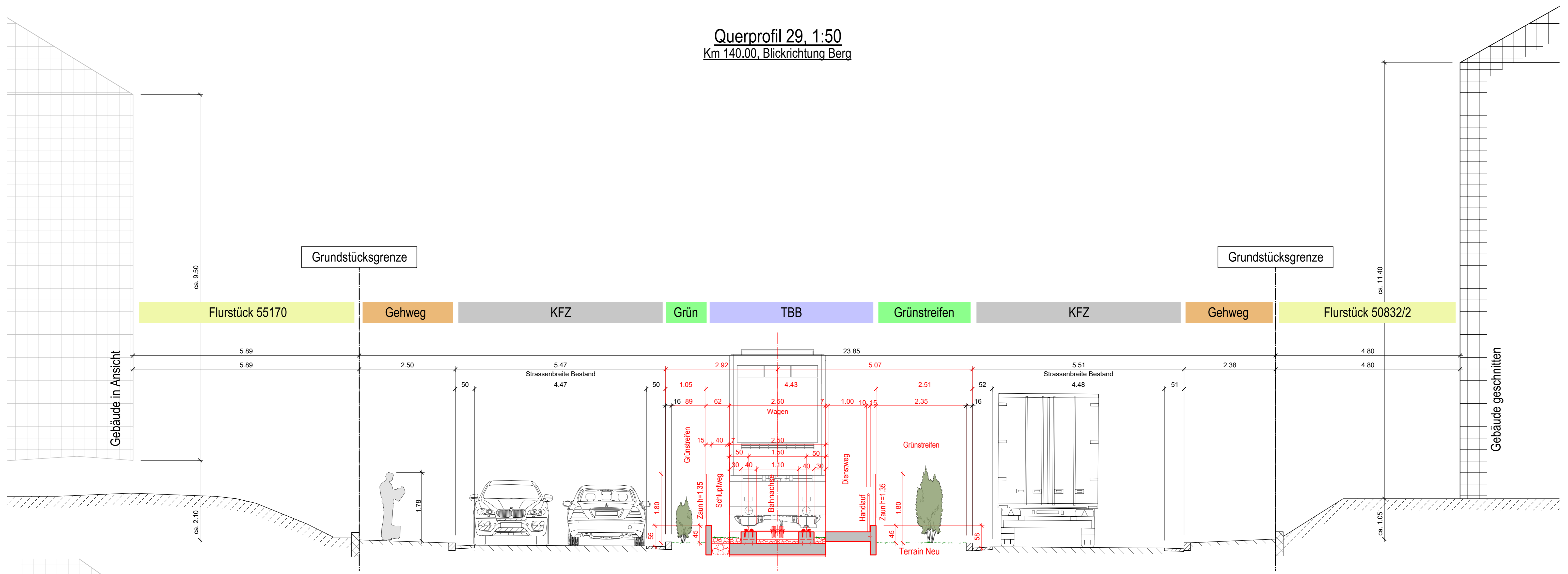
Querprofil 20, 1:50 Km 95.00, Blickrichtung Berg
